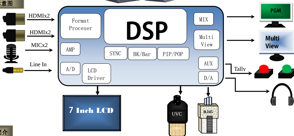
功能示意图
