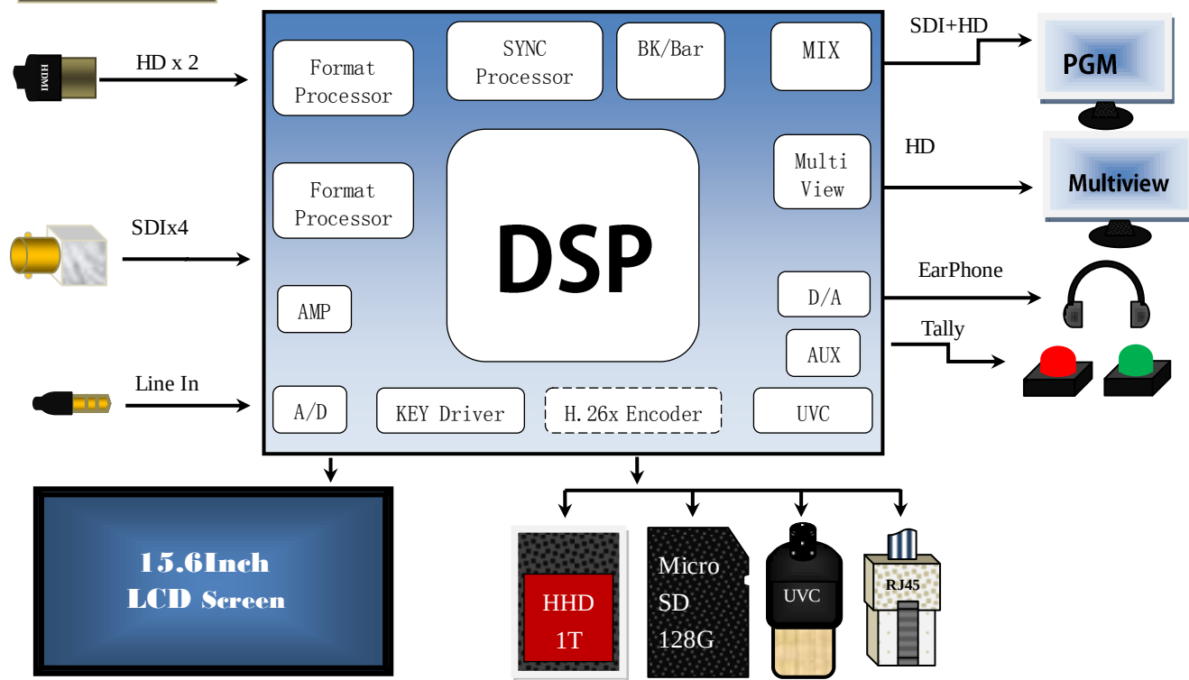
功能示意图
